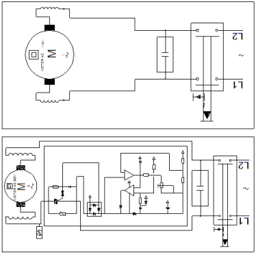
ESQUEMA ELECTRICO 110V 230V
