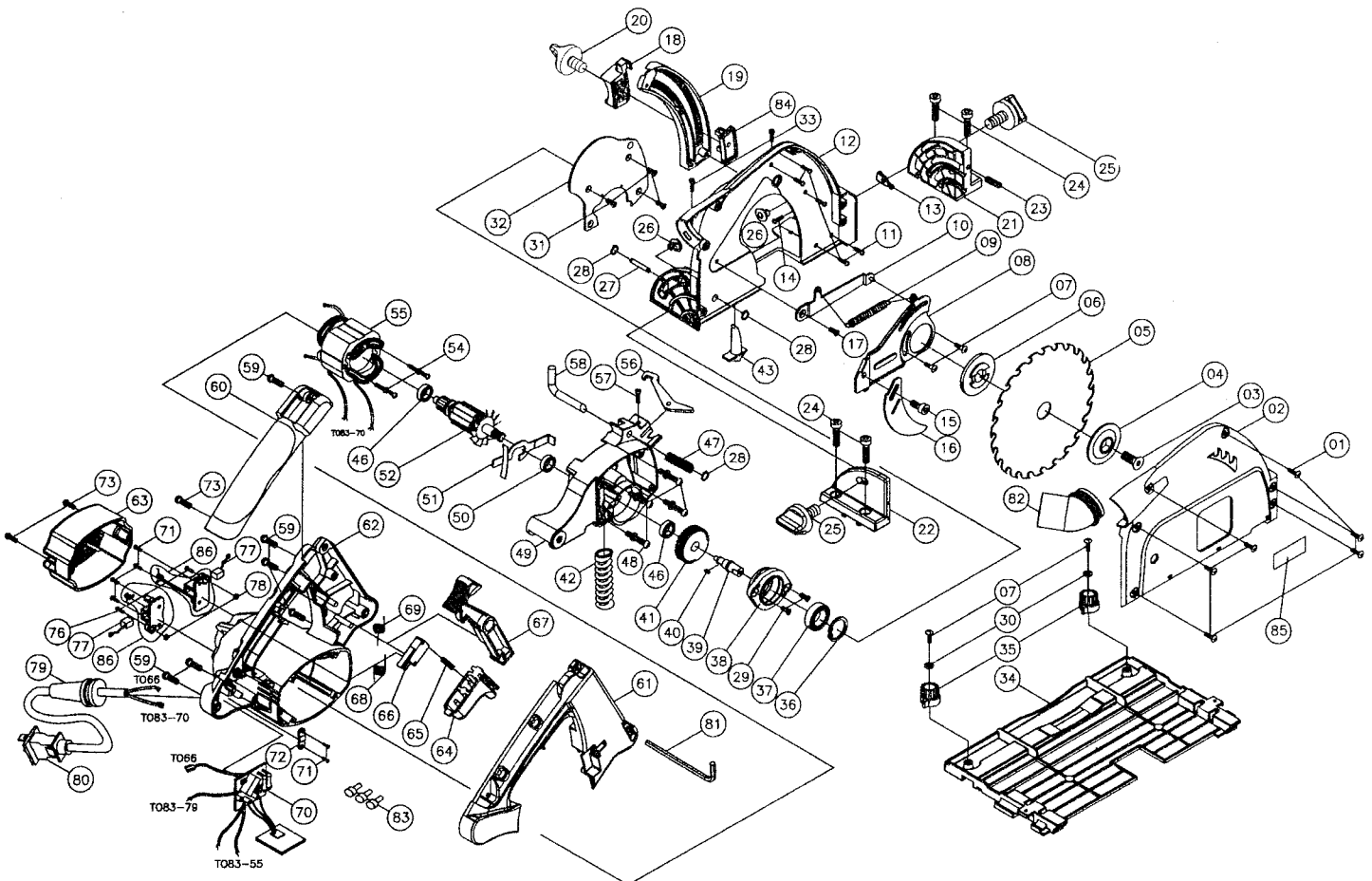
PLANO DESPIECE - 090909B
